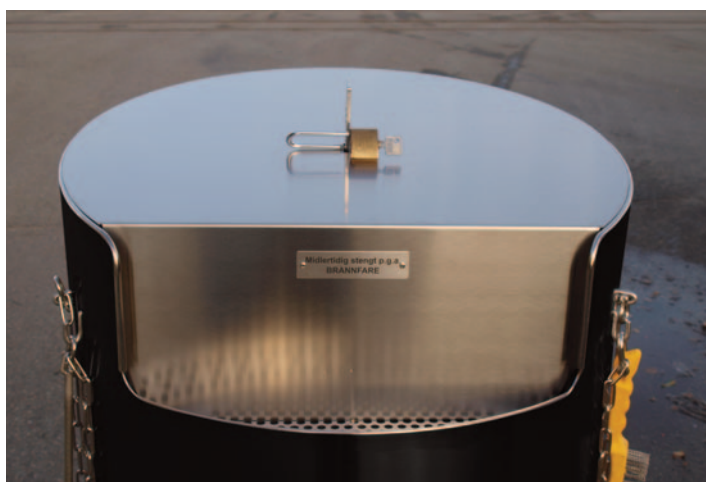
Avstengningsdeksel – ved fare for skog- eller gressbrann.
